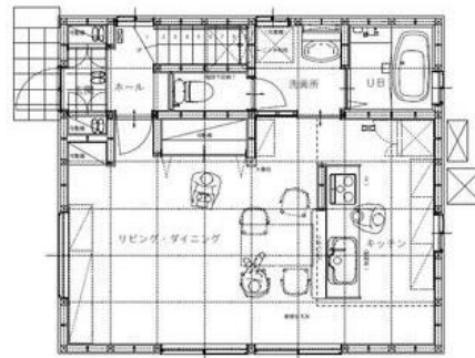
【1階】
